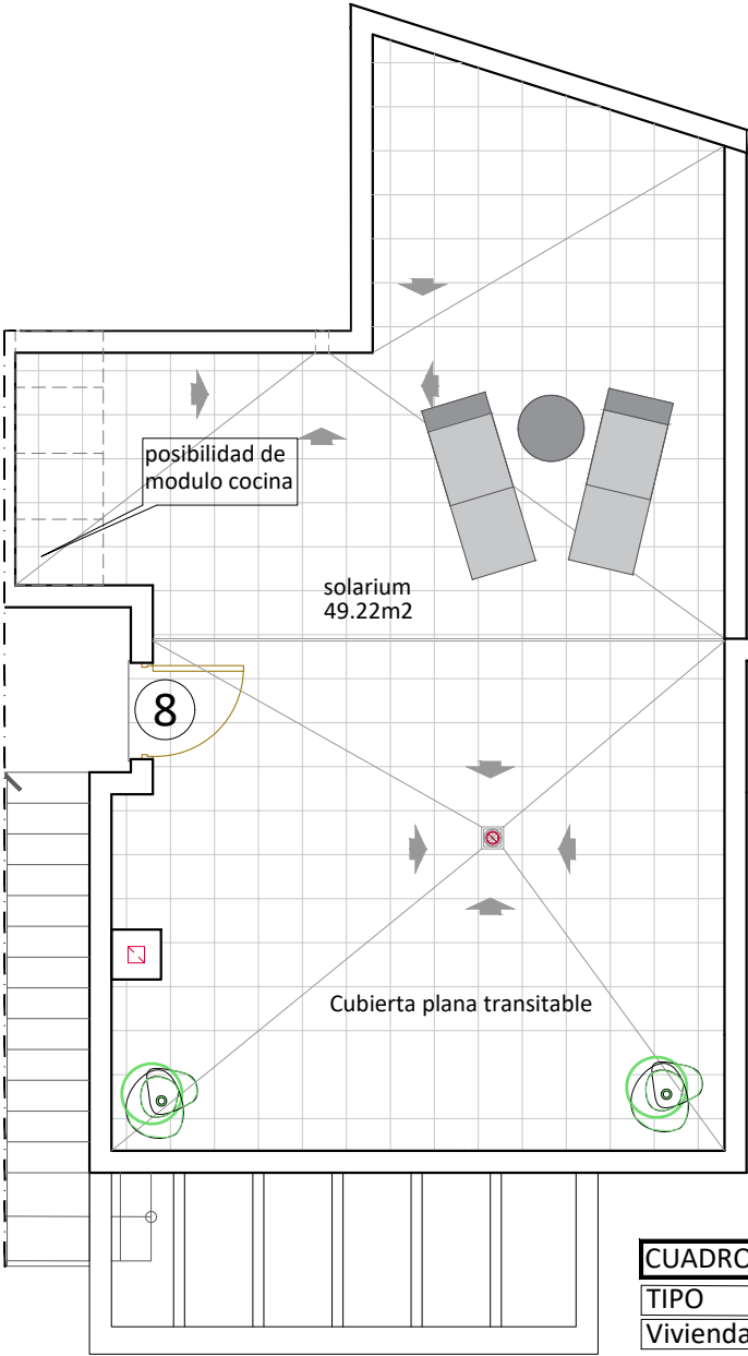
PLANTA SOLARIUM
