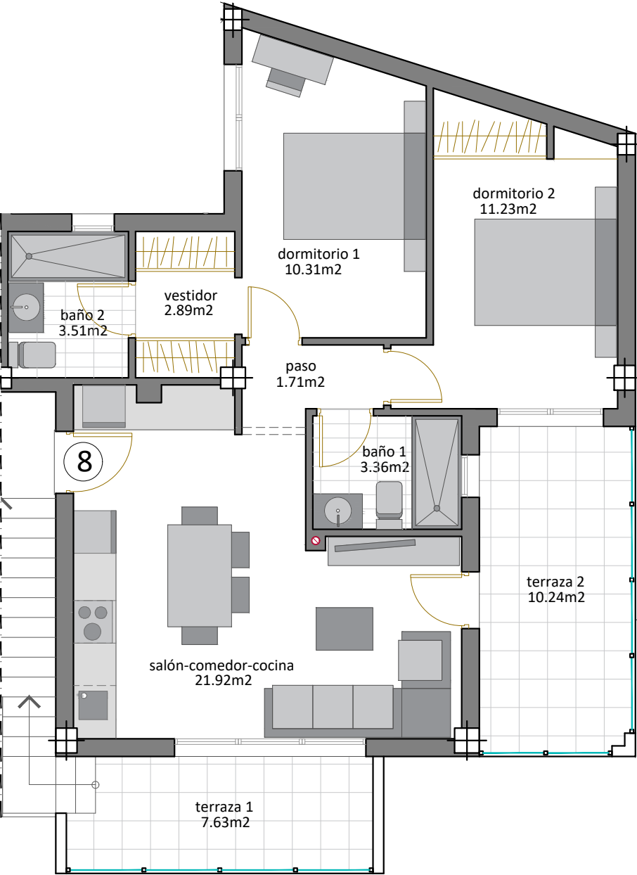
PLANTA PRIMERA
