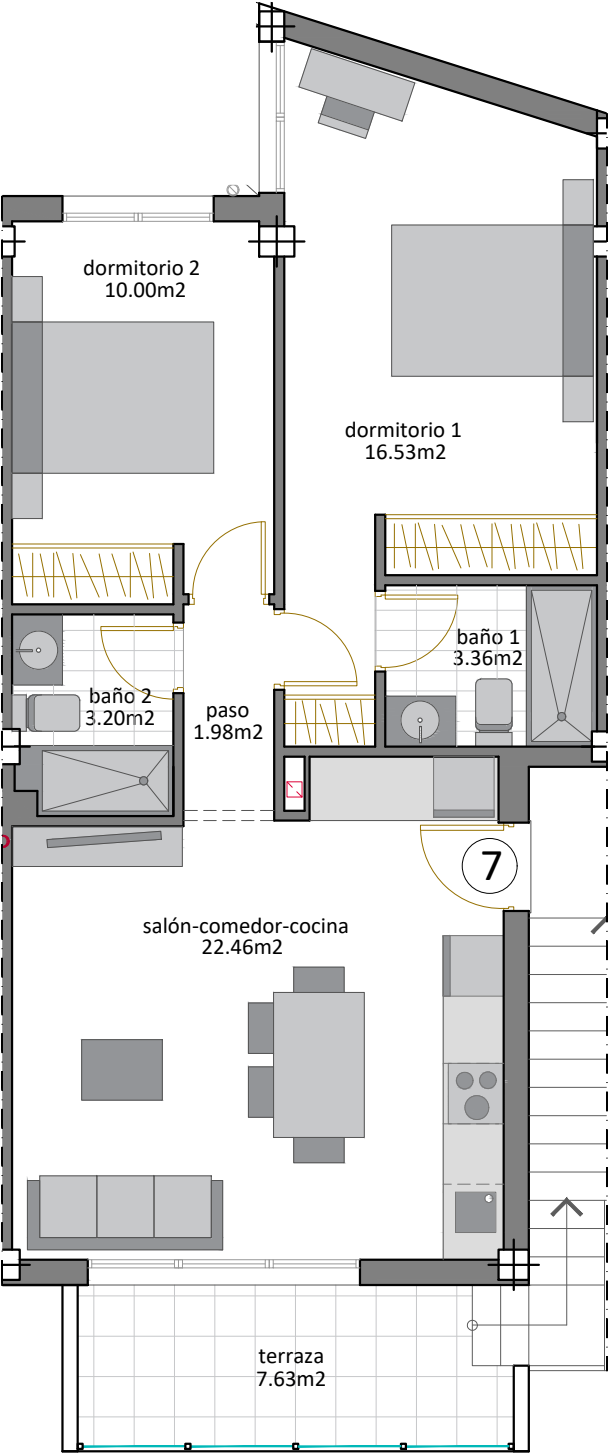
PLANTA PRIMERA
